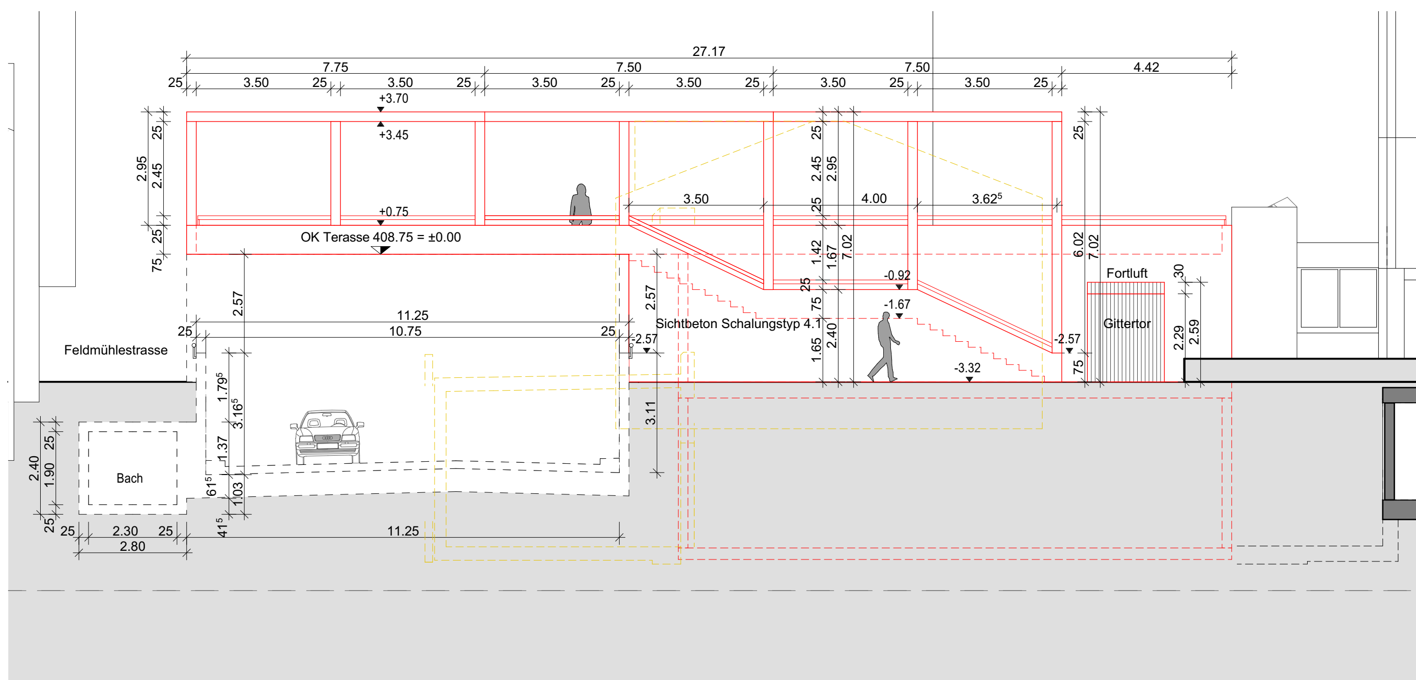
ANSICHT NORD
